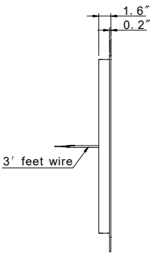
LEFT SIDE
